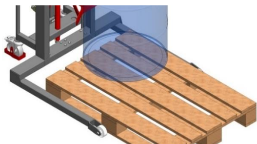
Modèle en longerons encadrant
