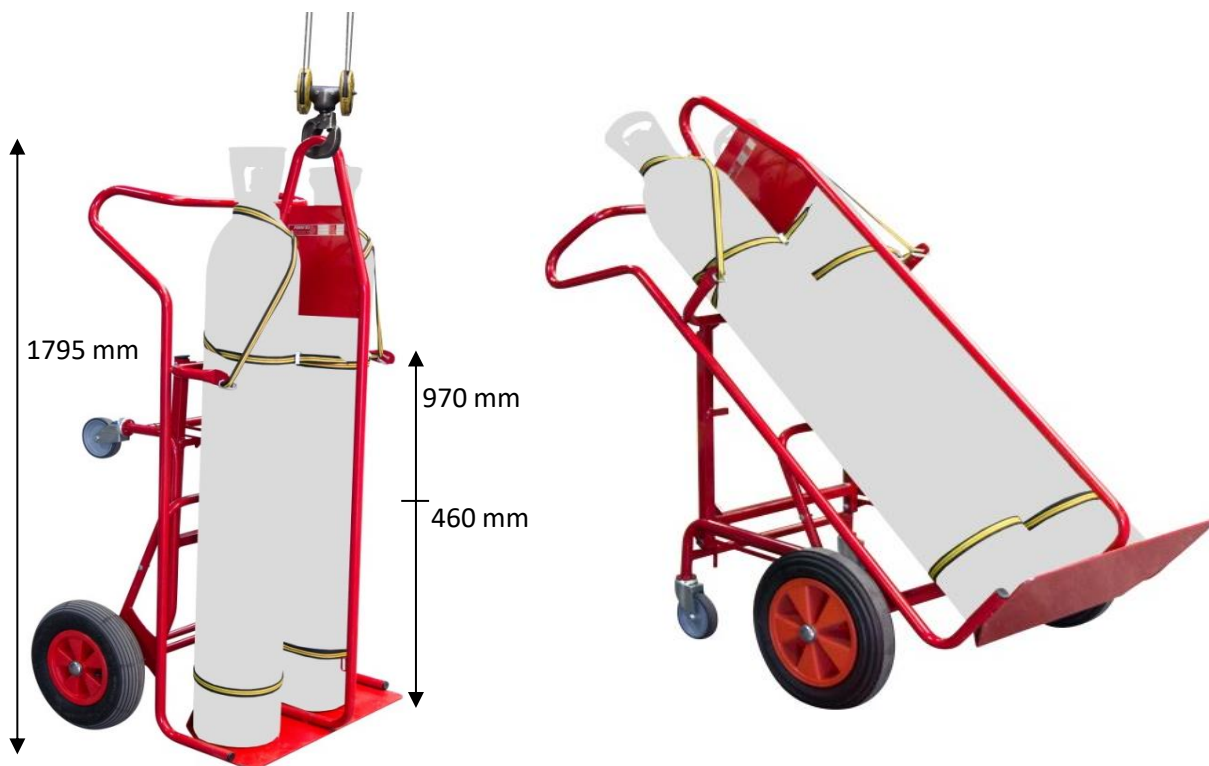
Diable élingable 2 bouteilles avec béquille
